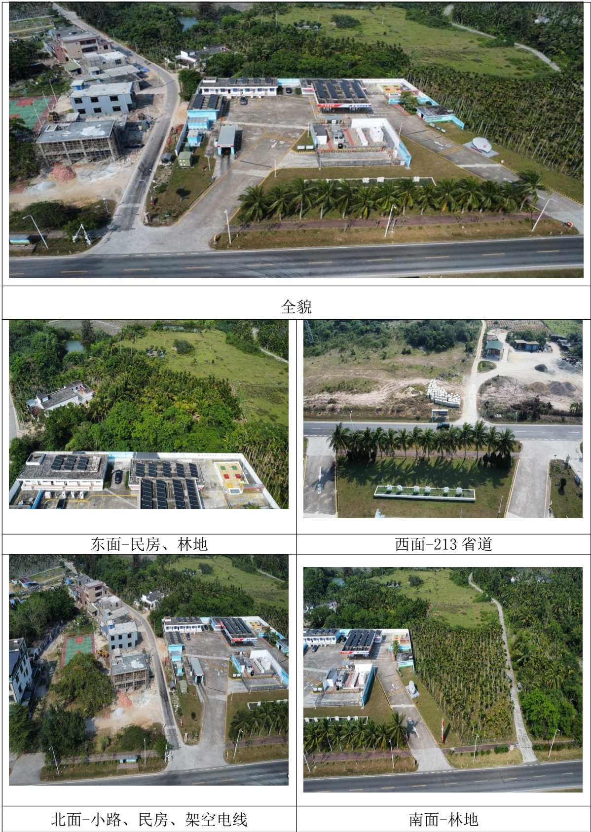
图 2.5-1 周边现状图
