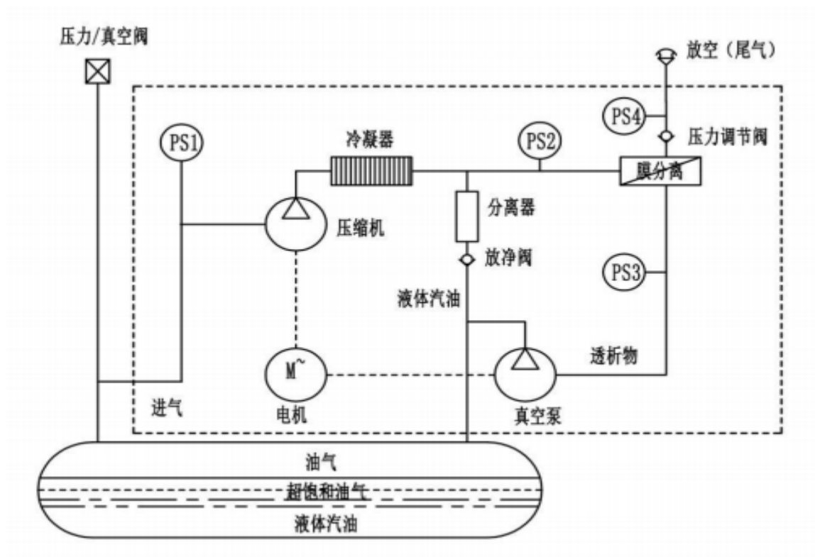
图 2.3-5 三次油气回收工艺流程图
