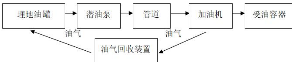
图 2.6-3 汽油加油工艺流程图
