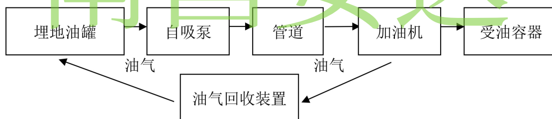
图 2.6-4 汽油加油工艺流程图
