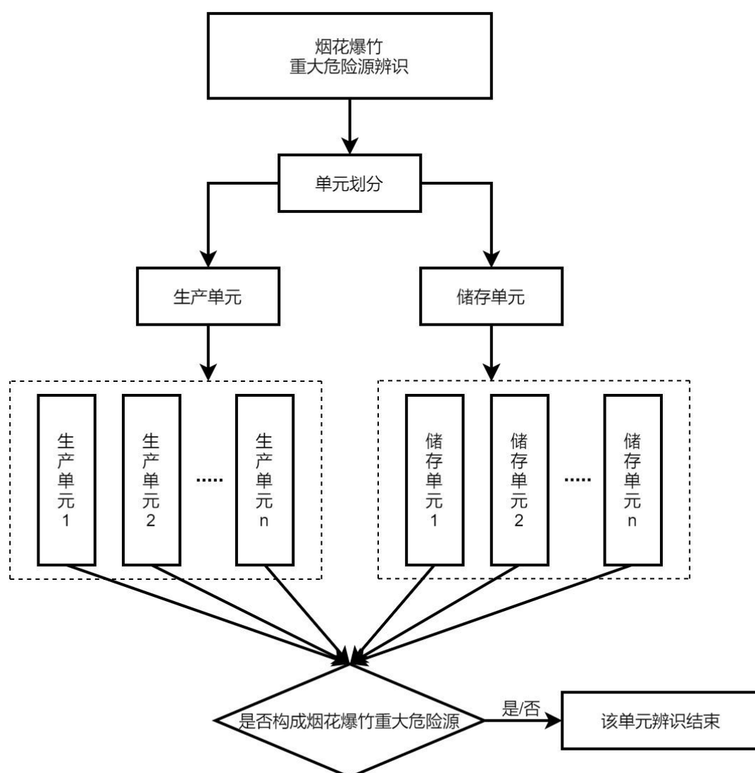
图 3.6-1 烟花爆竹重大危险源辨识流程图
