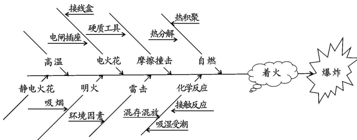
图 3.3-1 烟花爆竹引爆的因果分析图
