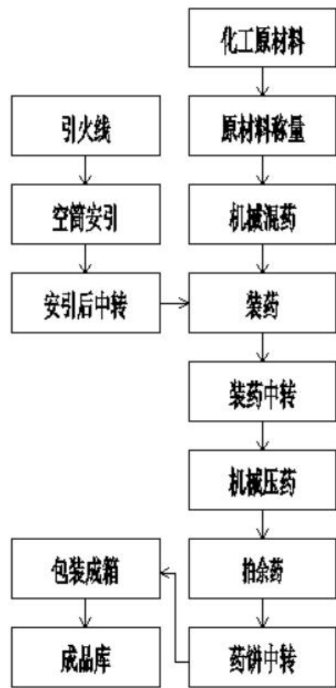
图 2-1：升空类（小火箭）生产工艺流程图
