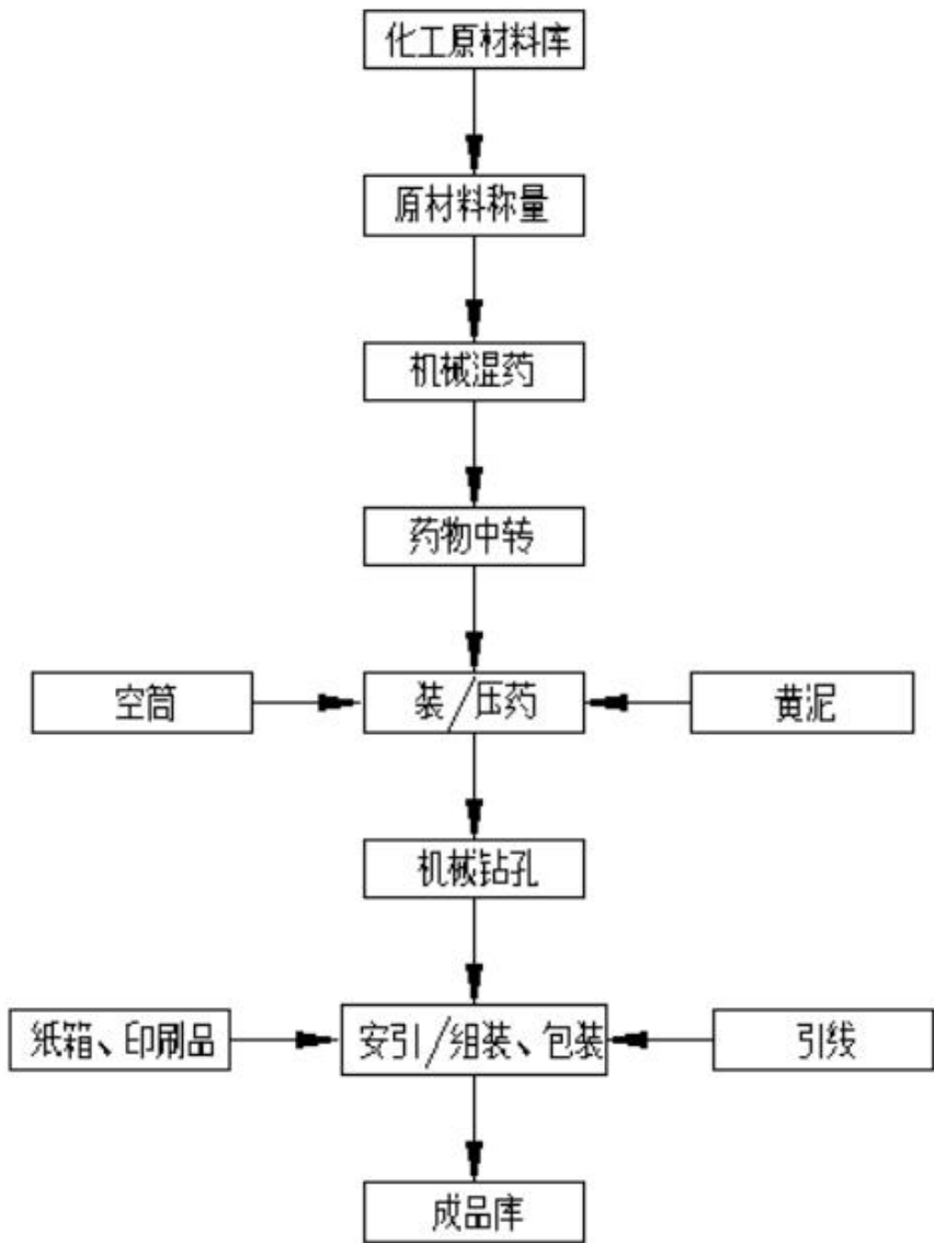
图 2-5：旋转类、升空类（旋转升空烟花）生产工艺流程图
