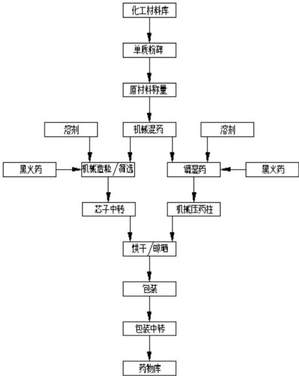
图 2-2：烟火药（亮珠/药柱）生产工艺流程图
