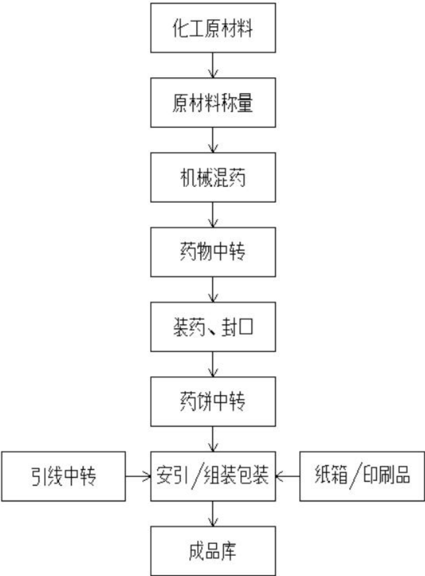
图 2-6：喷花类、玩具类（玩具造型）生产工艺流程图
