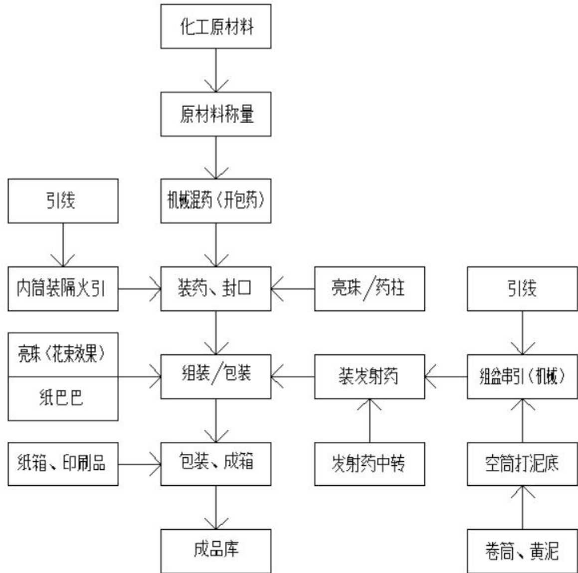
图 2-8：组合烟花类生产工艺流程图
