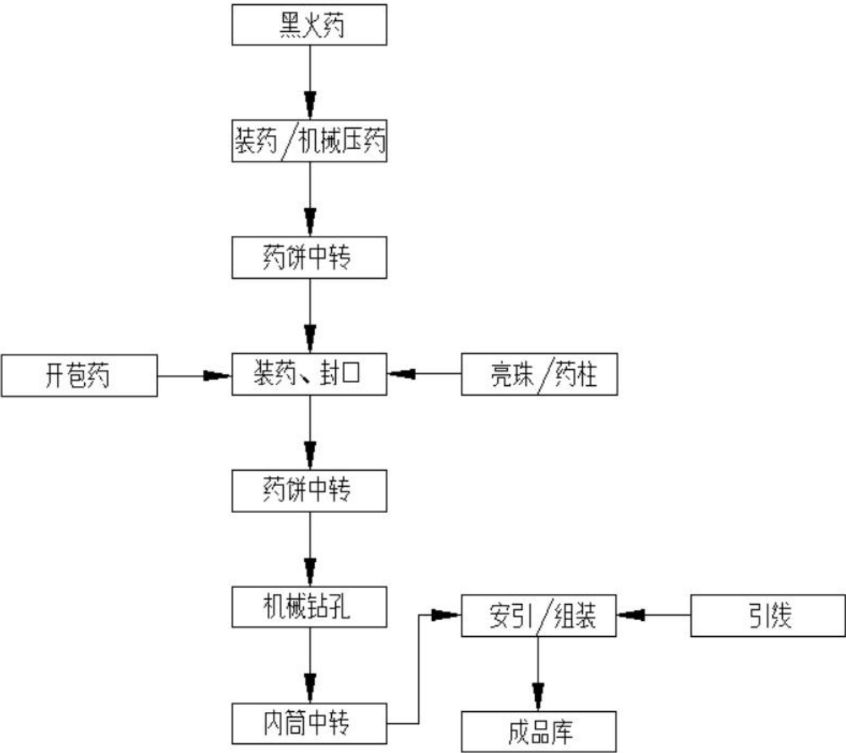
图 2-7：升空类（火箭、旋转升空烟花）生产工艺流程图
