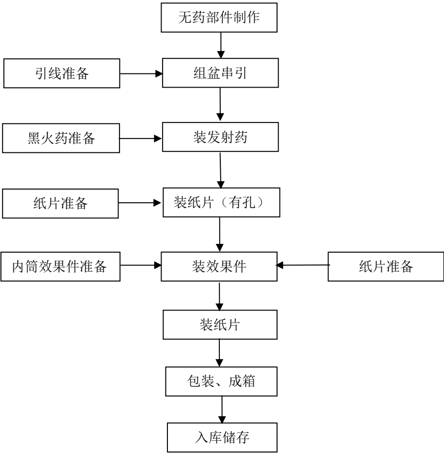
图 2.4-3 组合烟花类产品生产工艺流程图
