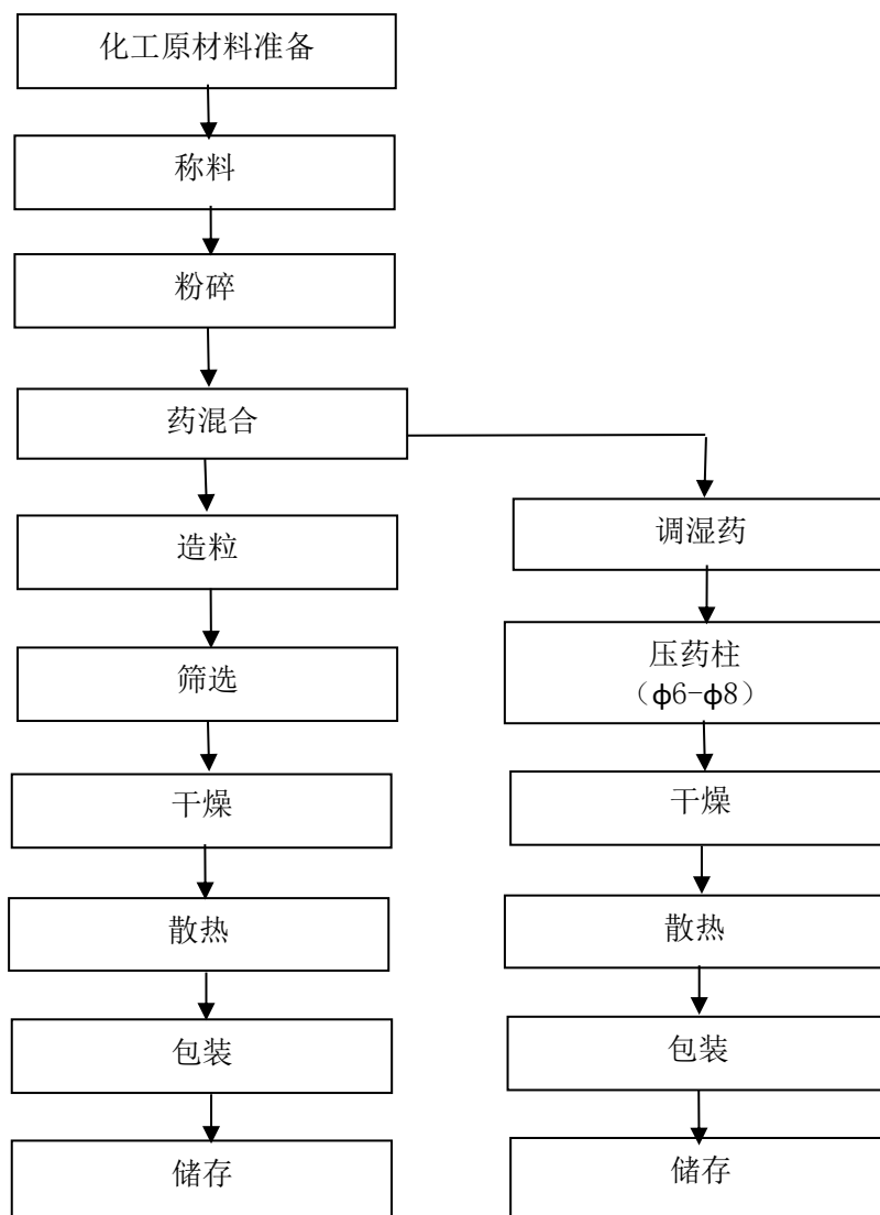
图 2.4-1 亮珠、药柱生产工艺流程图
