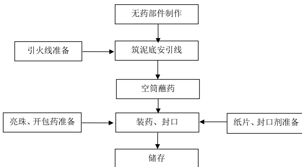
图 2.4-2 效果内筒生产工艺流程图
