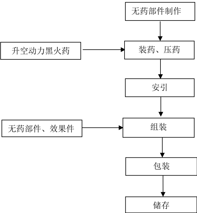
图 2.4-3 升空类（火箭）产品生产工艺流程图
