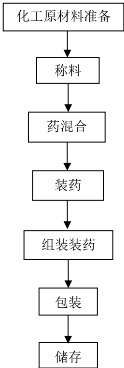
图 2.4-2 组合烟花类（飞天鼠）产品生产工艺流程图
