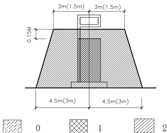
图 F3.3-3 汽油加油机爆炸危险区域划分
