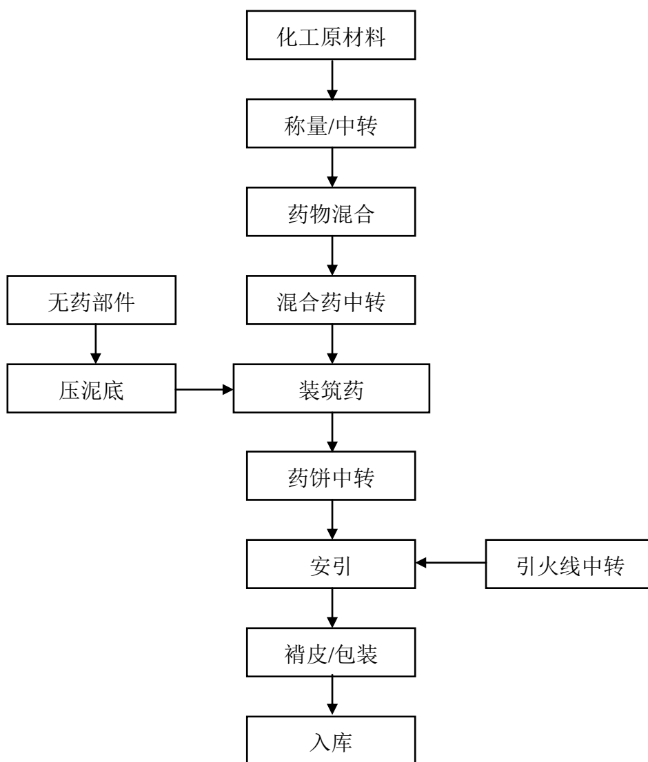
图 2.3-1 喷花生产工艺流程图
