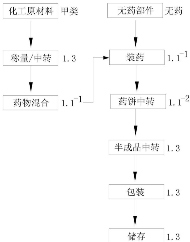
图2.3-4 线香类产品生产工艺流程图
