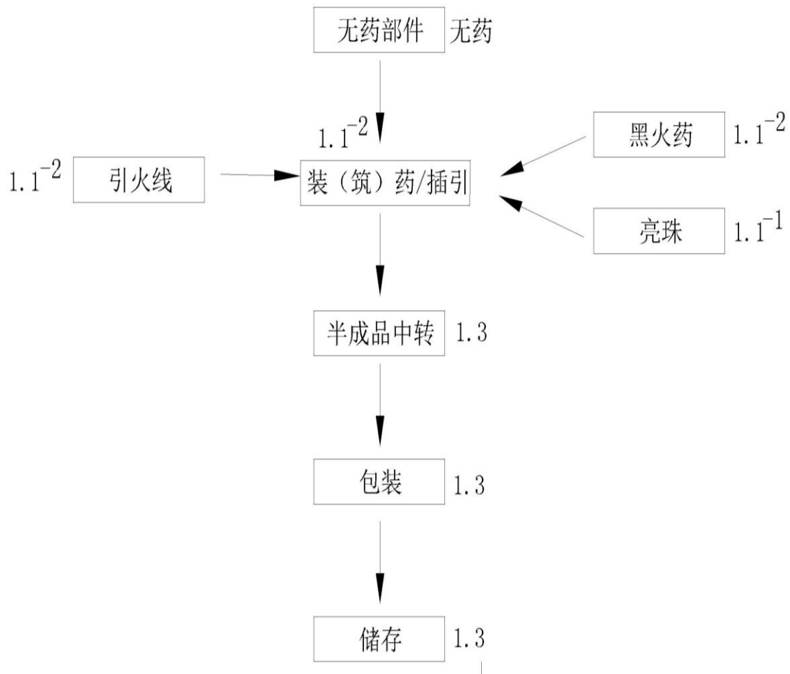
图 2.3-2 吐珠类产品生产工艺流程图
