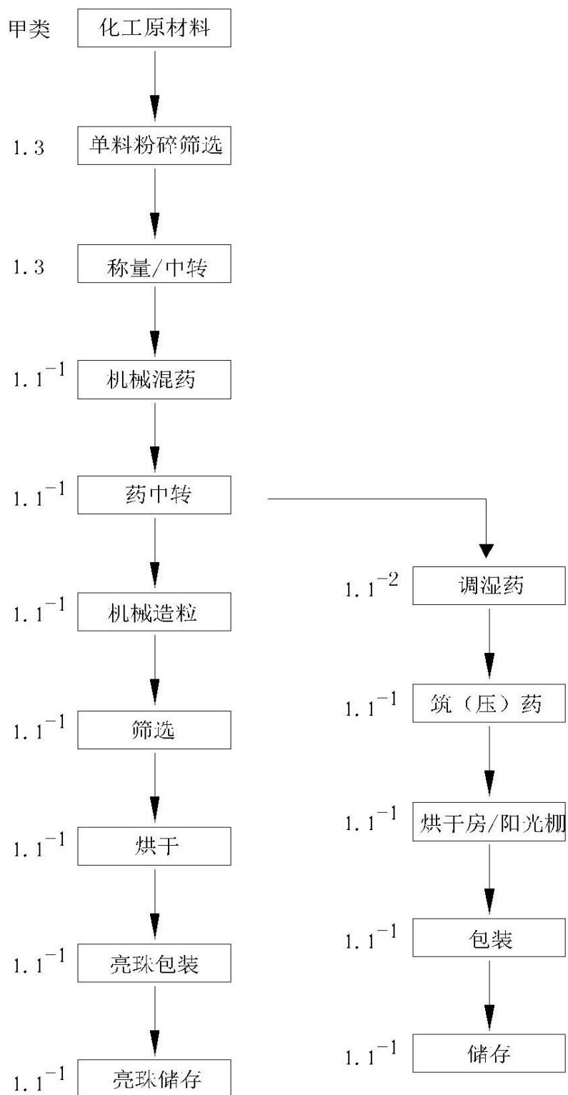
图 2.3-3 亮珠/药柱生产工艺流程图
