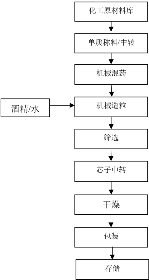
图 2-4：亮珠生产工艺流程图
