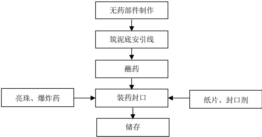
图 2-2：效果内筒生产工艺流程图
