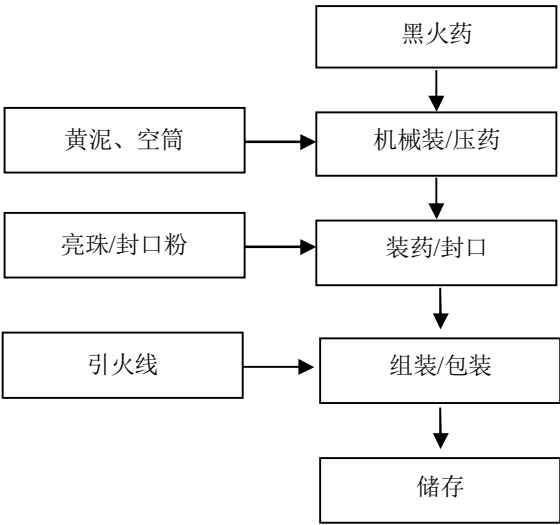
图 2-3：升空类（火箭）生产工艺流程图
