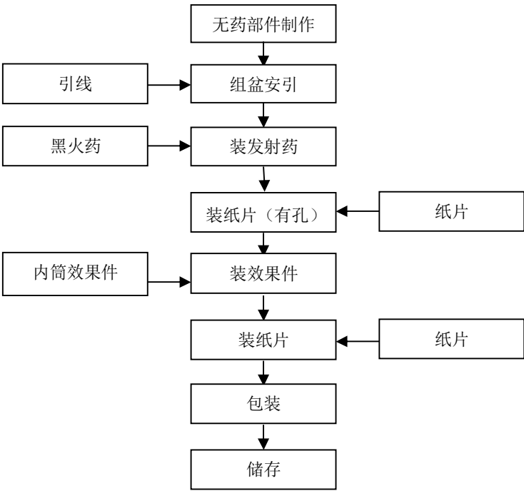
图 2-1：组合烟花生产工艺流程图
